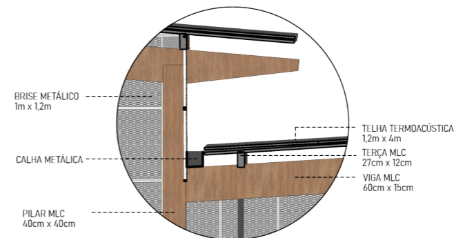
DET 01
