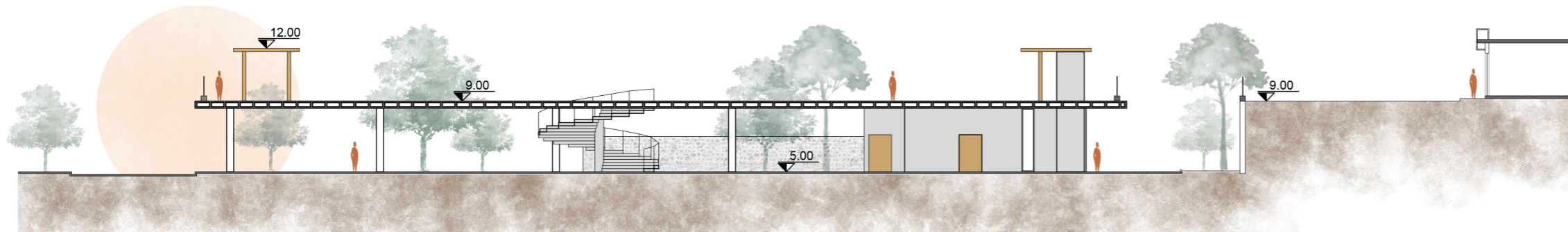
CORTE EE
