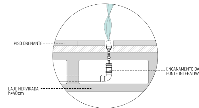
DET 04
