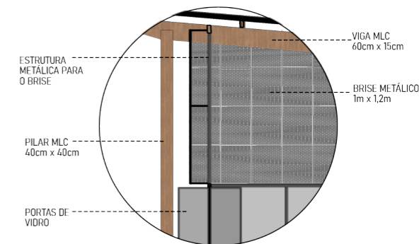
DET 02
