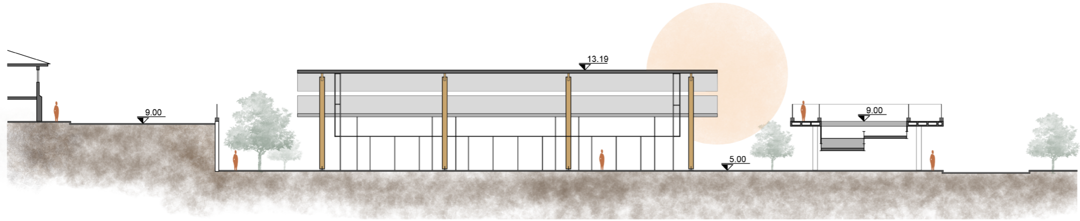
CORTE DD
