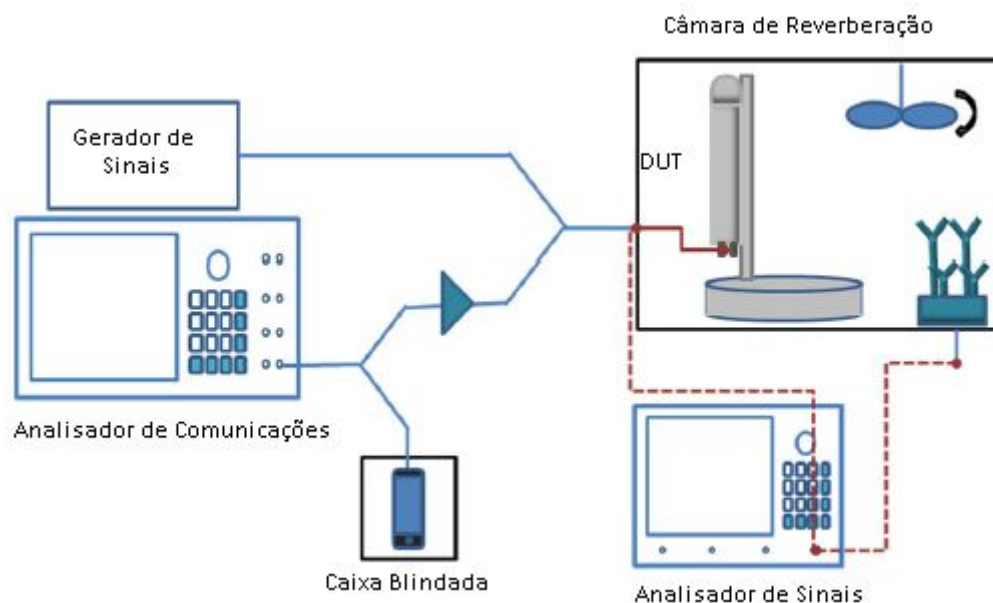
Figura 19 - Cenário de ensaio para medidas de ACLR
