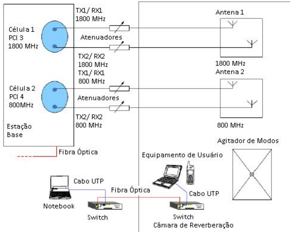
Figura 20 - Cenário de ensaio para medidas de Agregação de Portadoras
