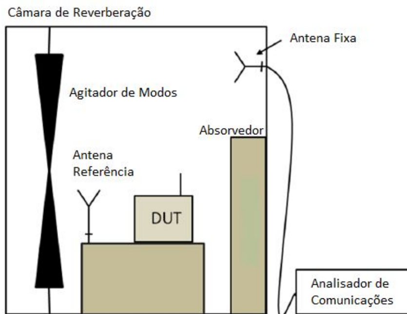
Figura 17 - Setup de ensaio para medições de TRP e TIS
