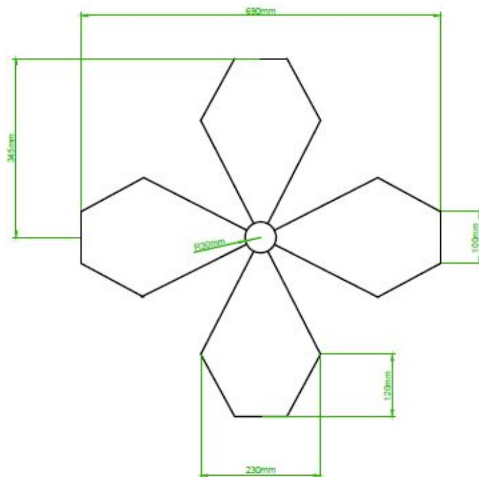
Figura 27: Agitador de Modos
